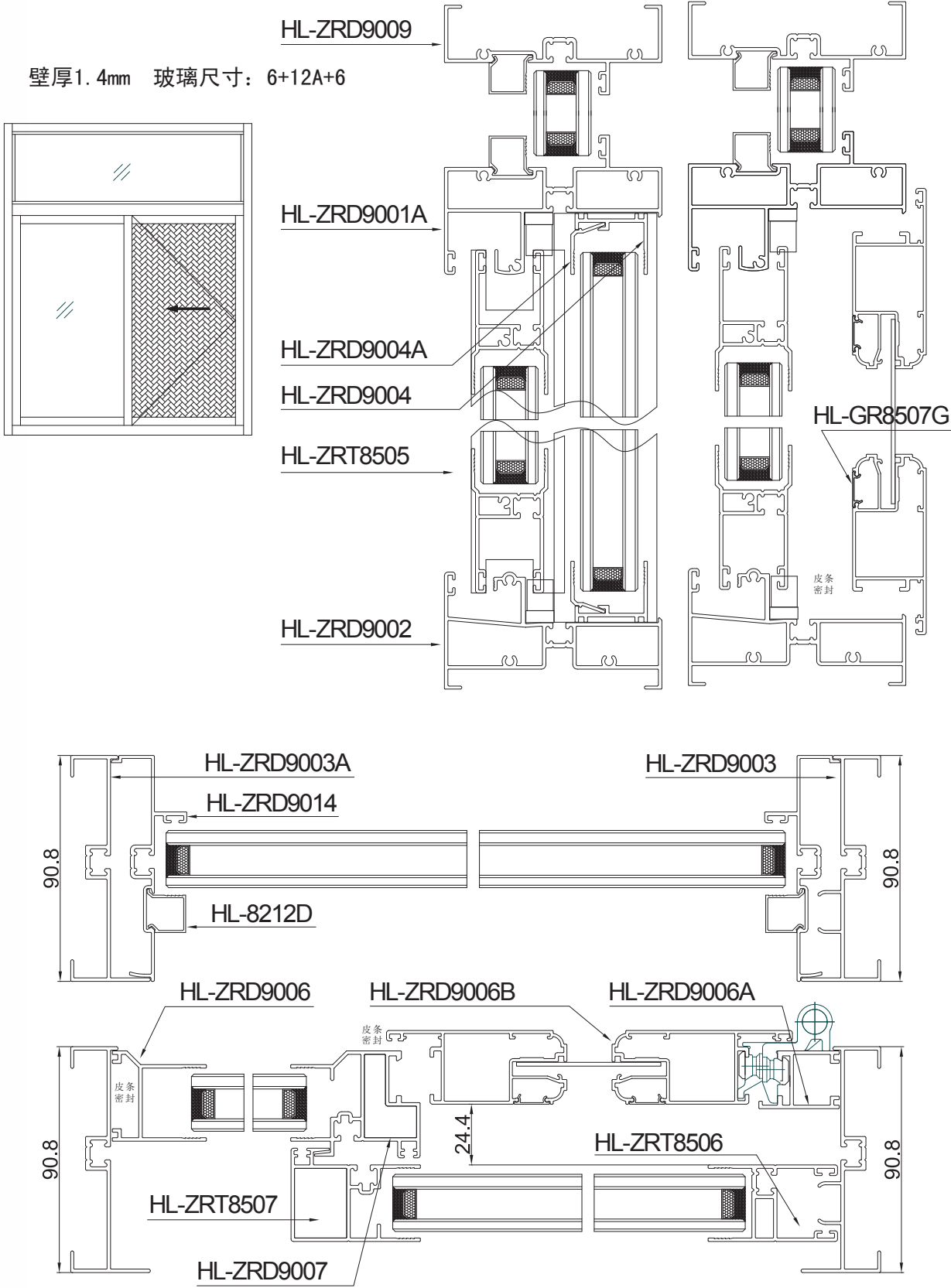
HL-注胶908单推拉系统窗
