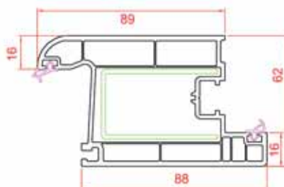
Door Sash
