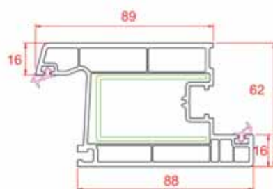
Door Sash
