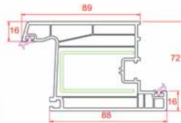
Door Sash
