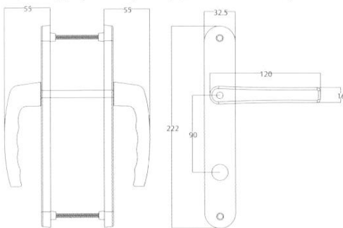
AKK16 Alüminyum WC Kapı Kolu FIRST Aluminium WC Door Handle FIRST Алюминиевая Дверная Ручка Для Ванной и Туалета FIRST
