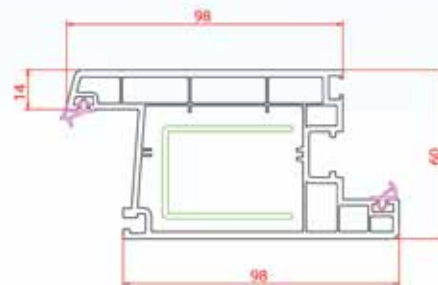
Door Sash
