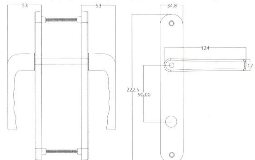
AKK17 Alüminyum WC Kapı Kolu YAKUT Aluminium WC Door Handle YAKUT Алюминиевая Дверная Ручка Для Ванной и Туалета YAKUT
