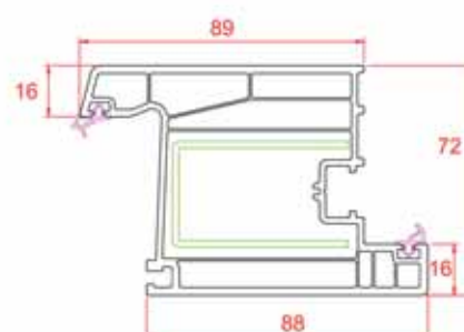
Door Sash
