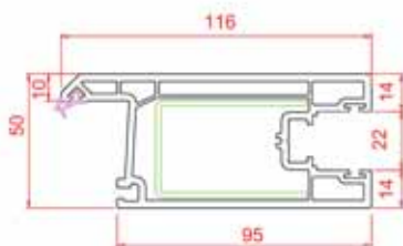
Door Sash
