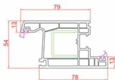
Door Sash
