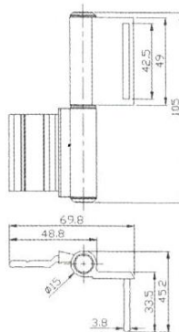
D. Aldoks Binme Menteşe D. Aldoks Series Hinge Петли для Алюминиевых Окон и Дверей
