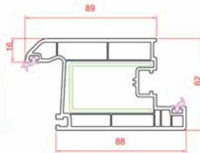
Door Sash
