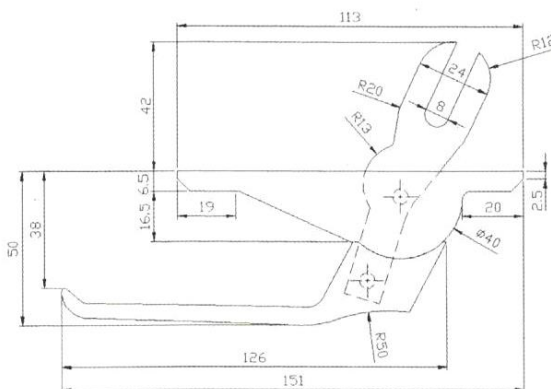
İspanyolet Kol - Klasik Espagnolette Handle - Classic Ручка для Алюминиевых окон
