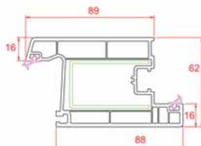
Door Sash
