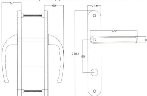
AKK19 Alüminyum WC Kapı Kolu Dar Ayna REKA Aluminium Wc Door Handle Narrow Type REKA Алюминиевая дверная ручка для ванна Узкая REKA
