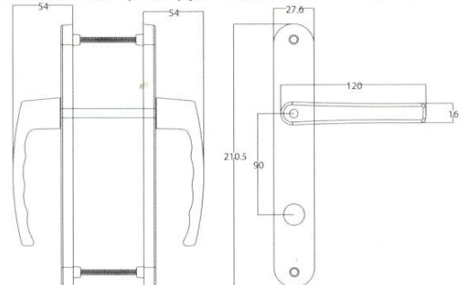
AKK22 Alüminyum WC Kapı Kolu Dar Ayna FIRST Aluminium Wc Door Handle Narrow Type FIRST Алюминиевая дверная ручка для ванна Узкая FIRST
