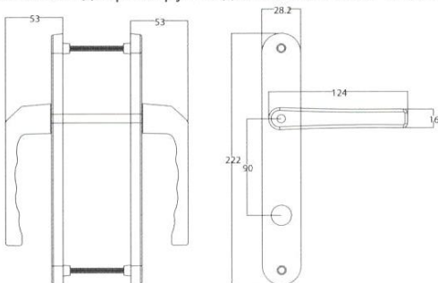
AKK21 Alüminyum WC Kapı Kolu Dar Ayna YAKUT Aluminium Wc Door Handle Narrow Type YAKUT Алюминиевая дверная ручка для ванна Узкая YAKUT
