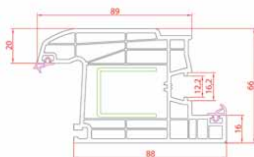
Door Sash
