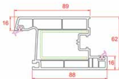
Door Sash
