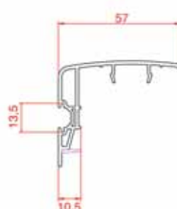
Interlock
