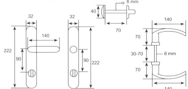
PLK03 Plastik WC Kapı Kolu KANARYA Plastic Door Handle WC KANARYA Пластиковая Дверная Ручка Для Ванной и Туалета KANARYA
