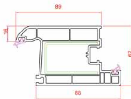
Door Sash
