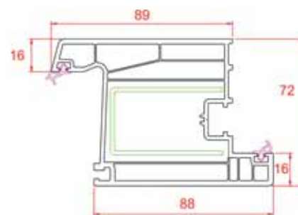
Door Sash
