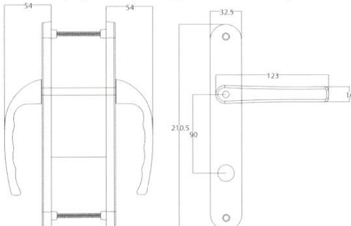
AKK18 Alüminyum WC Kapı Kolu REKA Aluminium WC Door Handle REKA Алюминиевая Дверная Ручка Для Ванной и Туалета REKA
